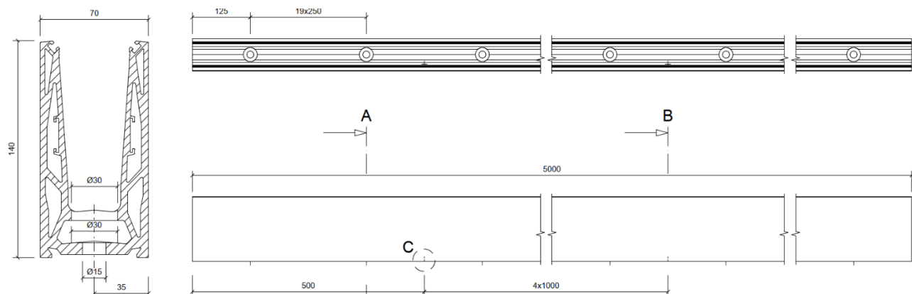
Abb. 1: Grundprofil U-Boden Aufsatzprofil
