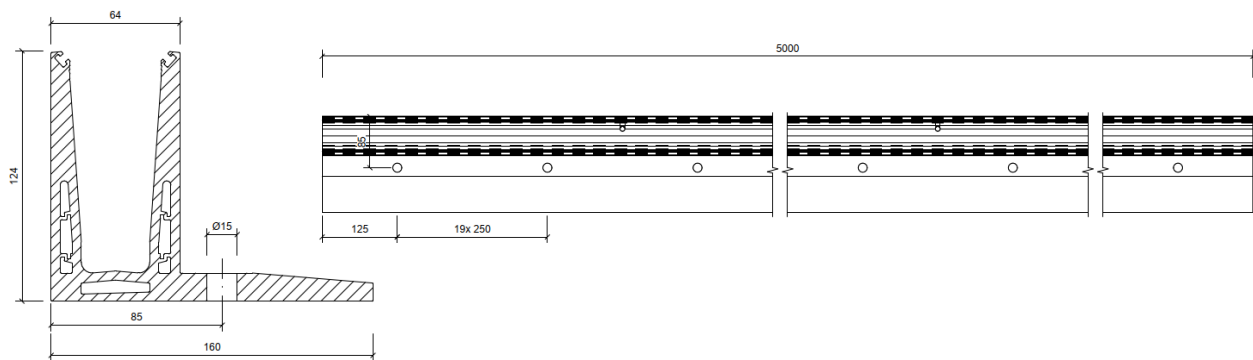
Abb. 3: Grundprofil V-Boden Aufsatzprofil
