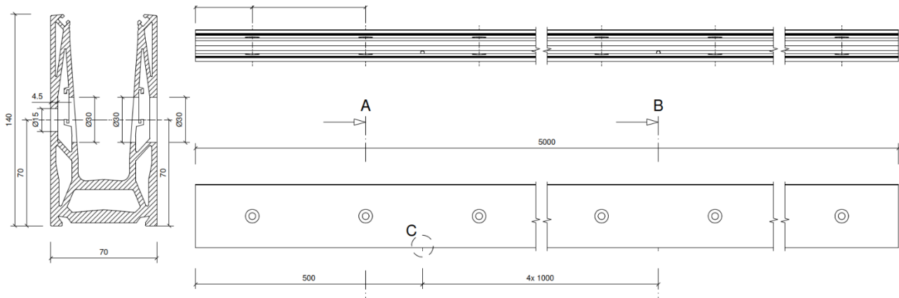
Abb. 2: Grundprofil U-Seitenprofil
