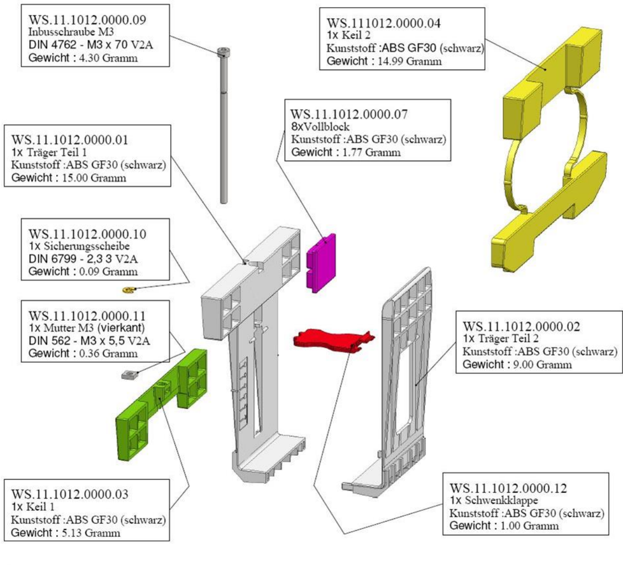
Abb. 5 Einzelkomponenten des Glasträgers
